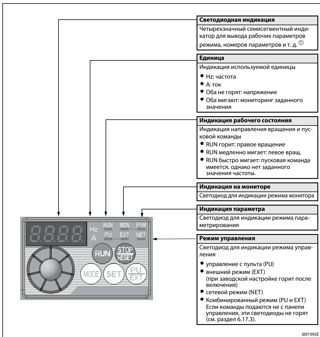
Рис. 4-6: Пульт управления преобразователя FR-D700 SC
