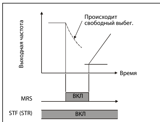
Рис. 6-43: Блокировка регулятора
