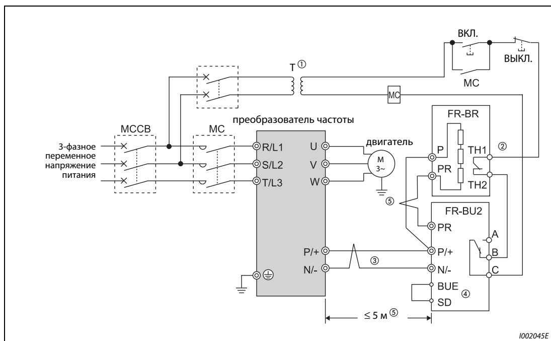
Рис. 3-31: Подключение тормозного блока типа FR-BU2
