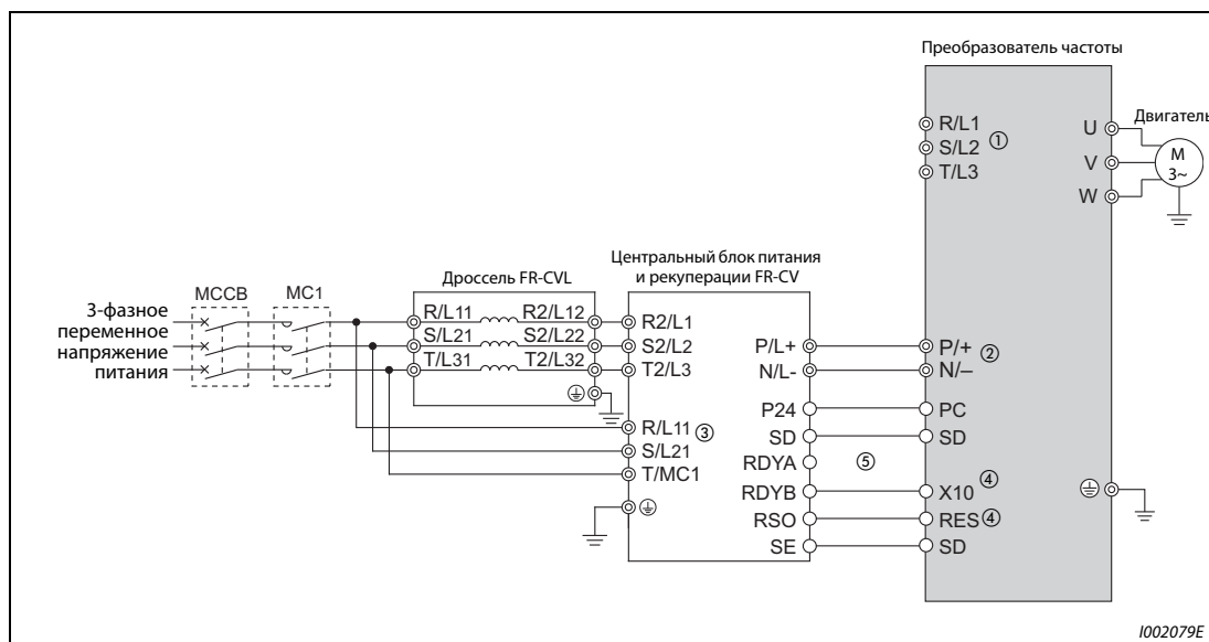
Рис. 3-33: Подключение комбинированного блока питания и рекуперации FR-CV
