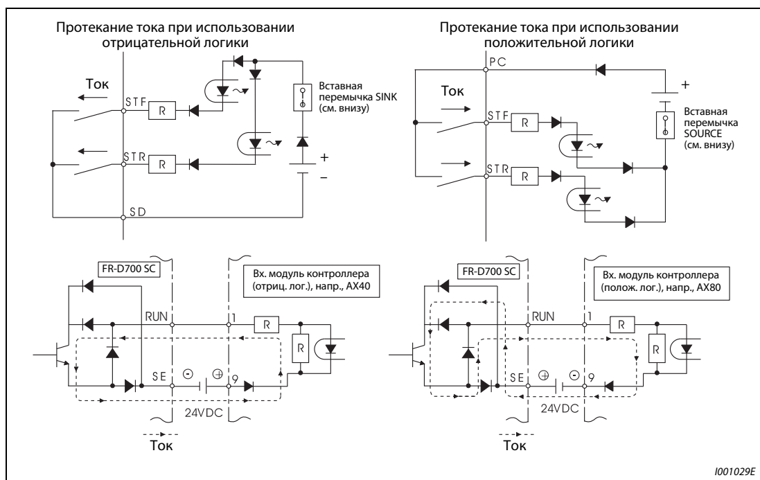
Рис. 3-17: Ток при отрицательной и положительной управляющей логике
