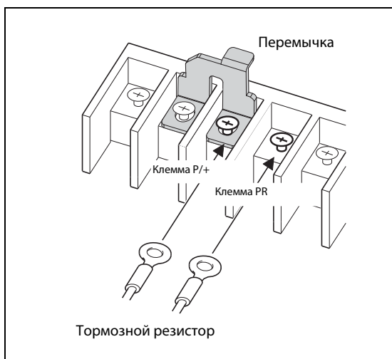
Рис. 3-26: Подключение тормозного резистора к клеммам P/+ и PR преобразователей частоты типов FR-D740-120SC и 160SC
