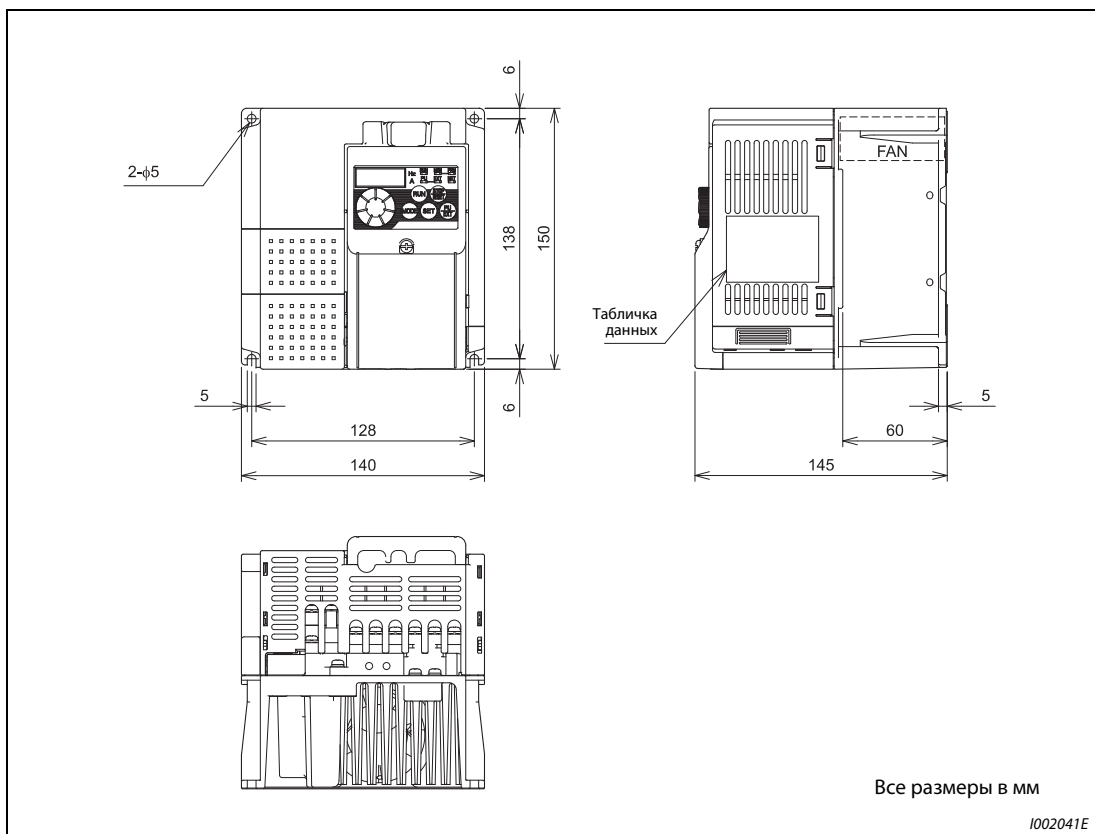
Рис. А-3: Размеры преобразователя частоты FR-D720S-100SC
