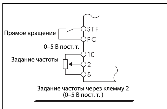
Рис. 6-80: Задание частоты в виде постоянного напряжения 0...5 В
