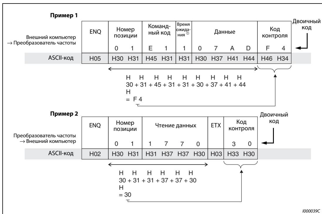
Рис. 6-111: Код контроля суммирования (примеры)
