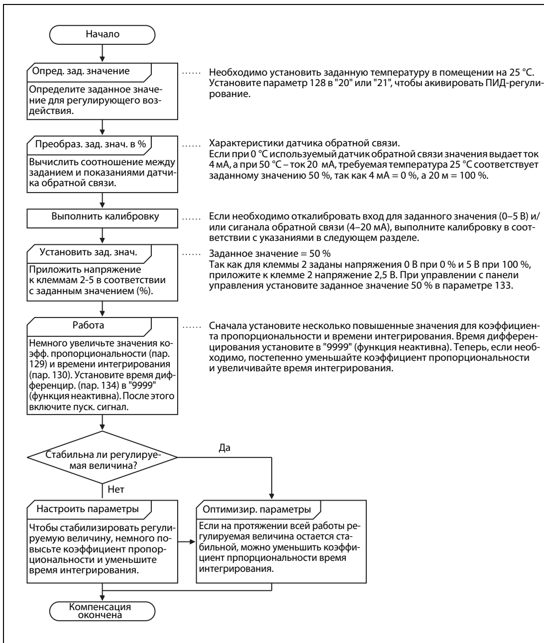
Рис. 6-129: Пример калибровки
