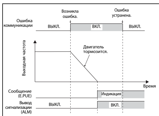
Рис. 6-107: Характер работы при пар. 502 = "1"
