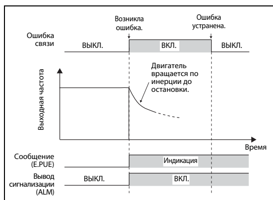
Рис. 6-106: Характер работы при пар. 502 = "0" (заводская настройка) или "3"
