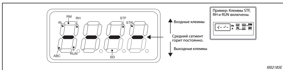
Рис. 6-62: Индикация коммутационных состояний клемм ввода/вывода
