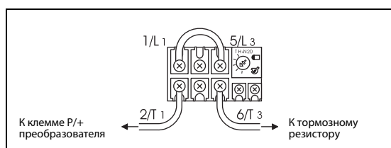
Таб. 3-19: Сочетание резистора и термореле
