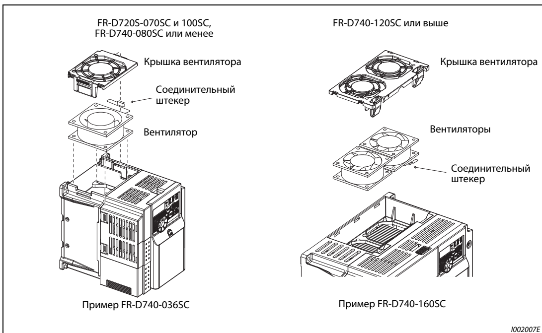
Рис. 8-3: Демонтаж вентилятора охлаждения
