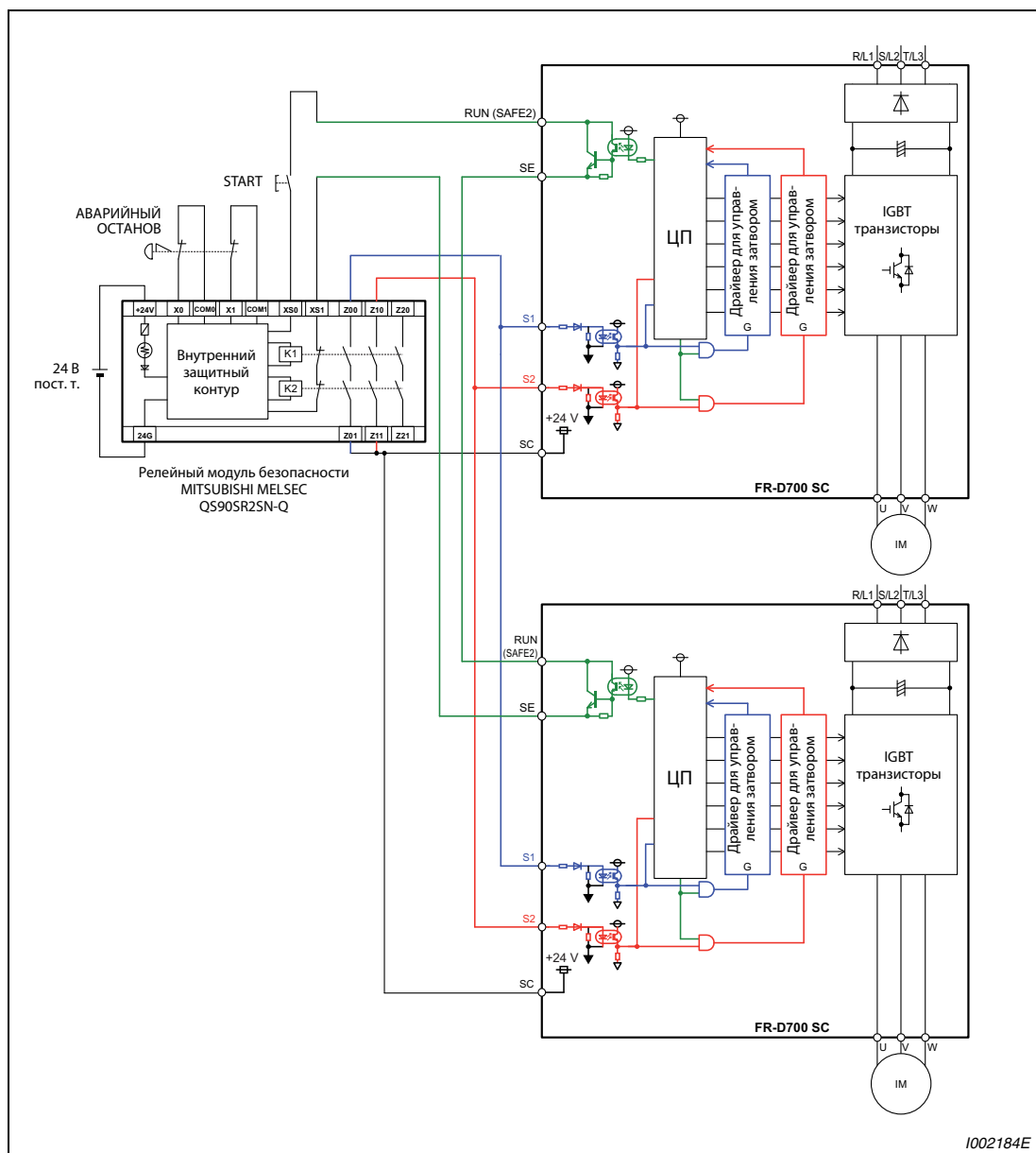
Рис. 3-16: Подключение нескольких преобразователей частоты к одному реле безопасности в случае применения функции "Безопасный останов"
