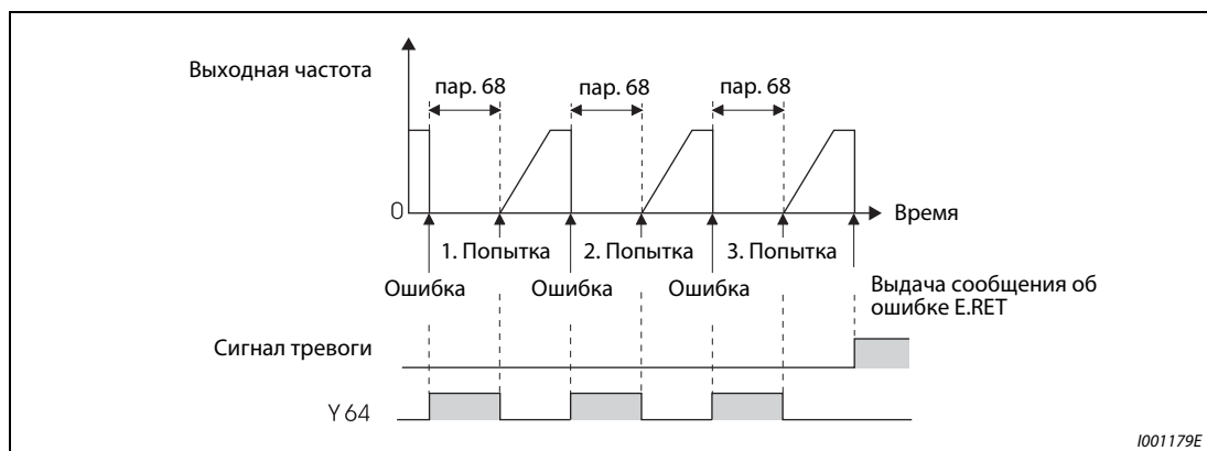
Рис. 6-77: Пример неудачных попыток перезапуска
