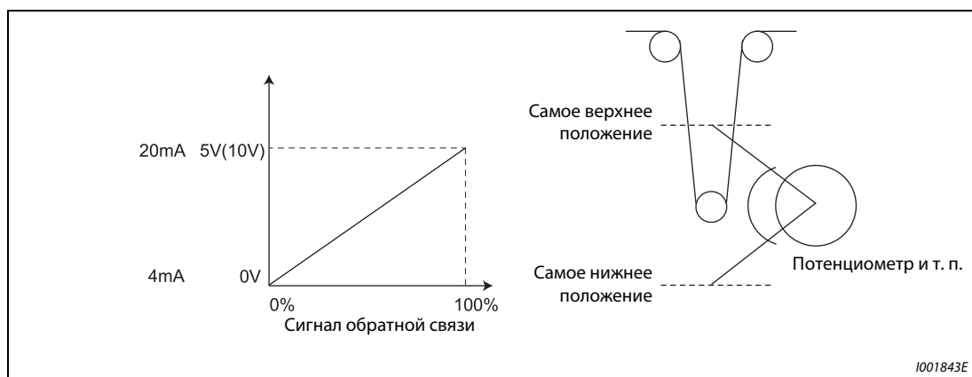
Рис. 6-135: Компенсация сигнала, характеризующего положение компенсирующего ролика
