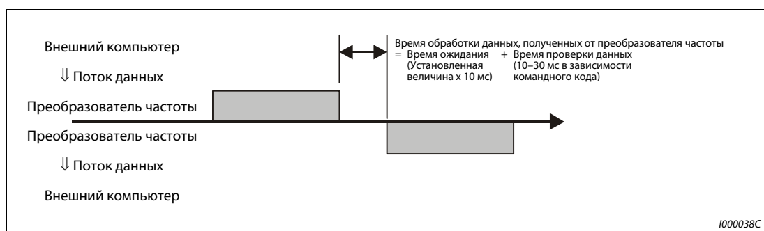
Рис. 6-110: Определение времени ожидания
