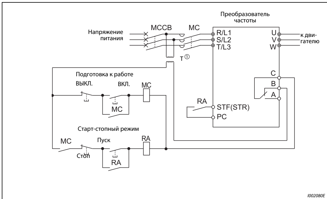
Рис. 3-23: Пример подключения преобразователя частоты
