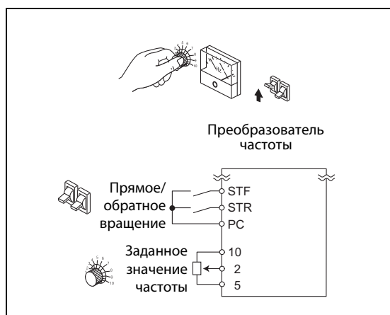
Рис. 6-92: Внешнее управление
