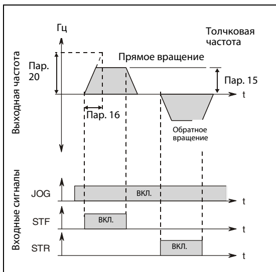
Рис. 6-19: Временная характеристика сигналов в толчковом режиме
