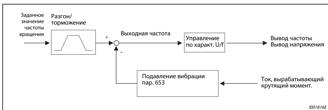
Рис. 6-78: Принцип подавления вибрации
