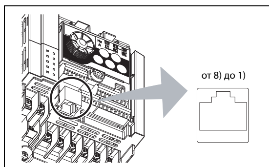
Рис. 6-96: Клеммы подключения панели управления (интерфейс PU)
