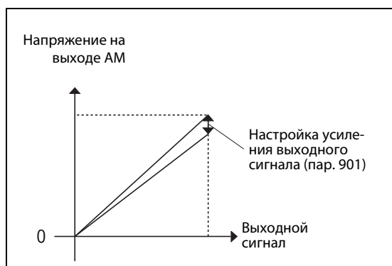
Рис. 6-66: Настройка усиления на выходе АМ
