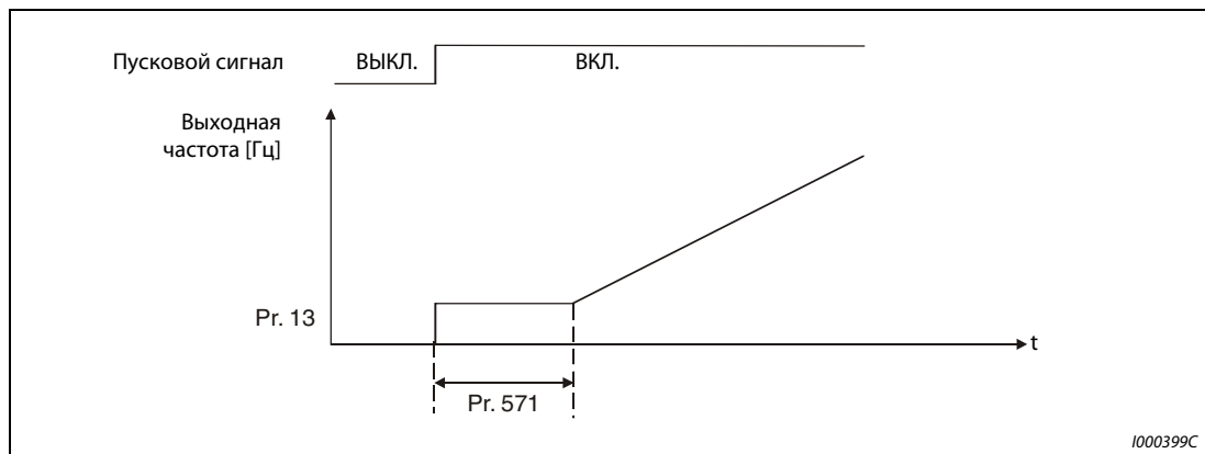
Рис. 6-29: Время удержания стартовой частоты
