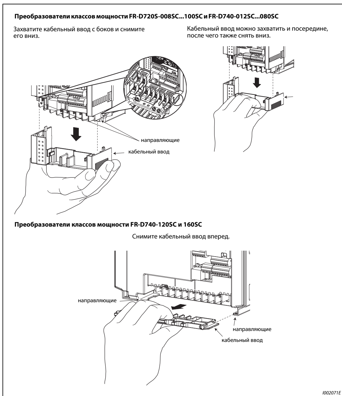
Рис. 2-5: Примеры удаления кабельного ввода
