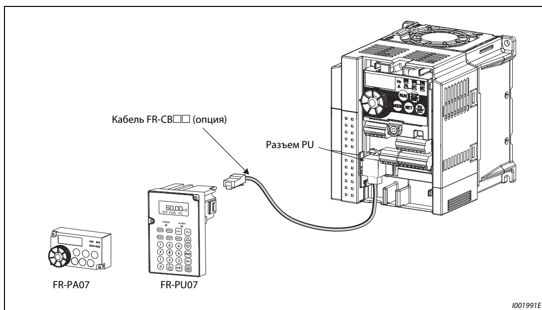
Рис. 3-22: Подключение пульта управления к интерфейсу PU
