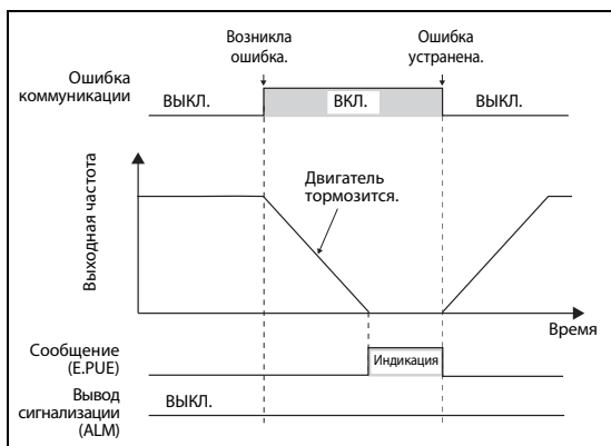
Рис. 6-108: Характер работы при пар. 502 = "2"
