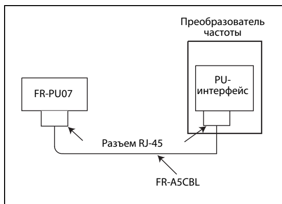
Рис. 6-97: Подключение пульта управления к интерфейсу PU
