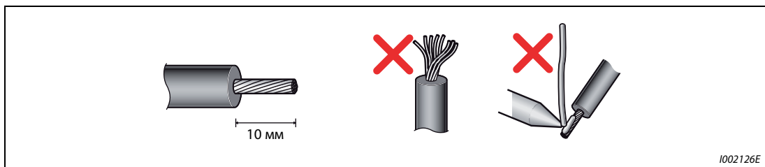
Рис. 3-7: Подготовка кабеля
