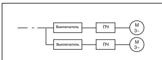
Рис. 3-2: Расположение силовых выключателей ("ПЧ" означает "преобразователь частоты")
