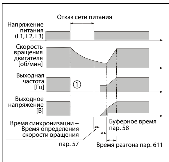
Рис. 6-69: Автоматический перезапуск с определением выходной частоты (пар. 162 = 0/10)
