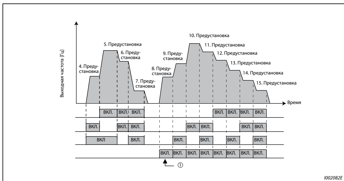
Рис. 6-16: Вызов предустановленных скоростей вращения в зависимости от наличия сигналов на клеммах
