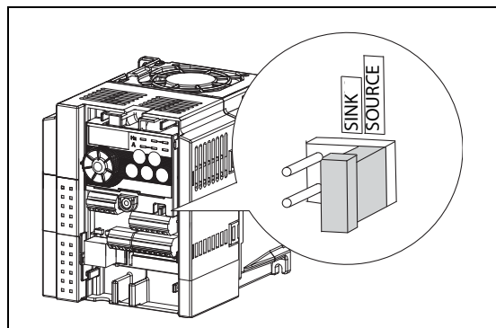
Рис. 3-18: Выбор логической схемы управления
