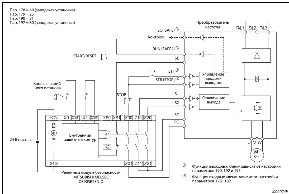
Рис. 3-15: Подключение релейного модуля безопасности Mitsubishi QS90SR2SN-Q
