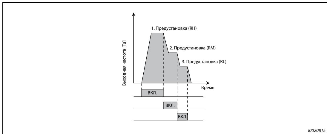
Рис. 6-15: Вызов предустановленных скоростей вращения в зависимости от наличия сигналов на клеммах
