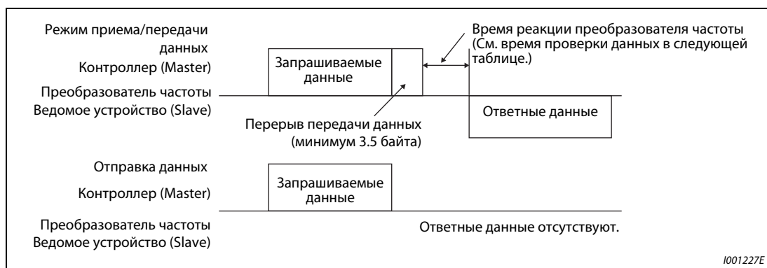
Рис. 6-116: Формат сообщений
