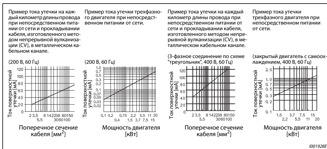
Рис. 3-37: Токи утечки
