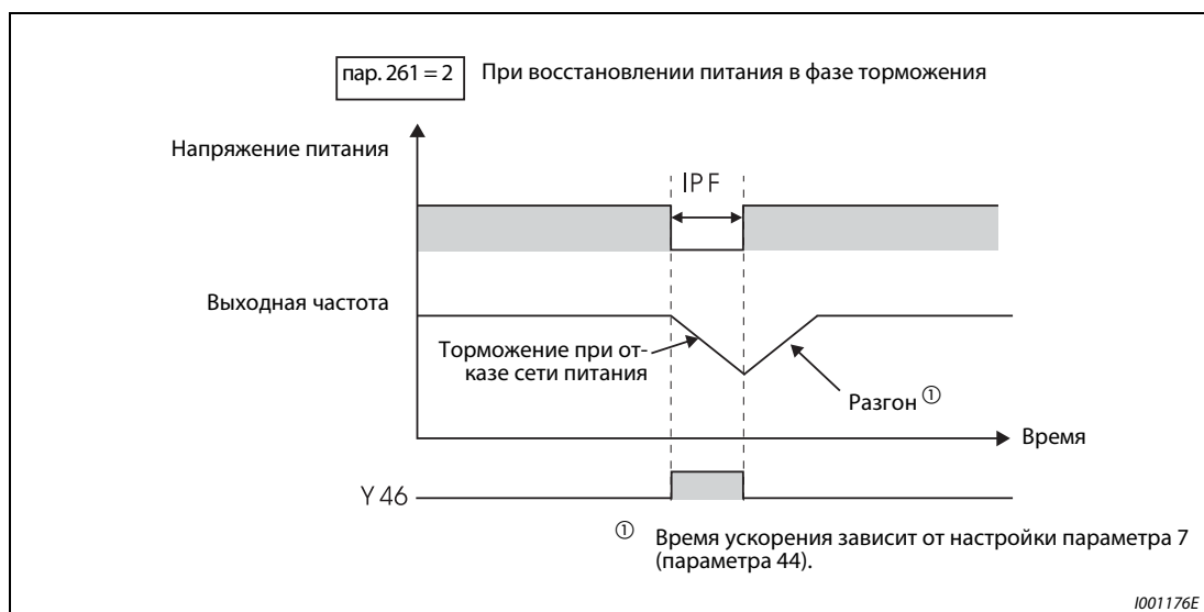
Рис. 6-74: Продолжение работы после отключения сети
