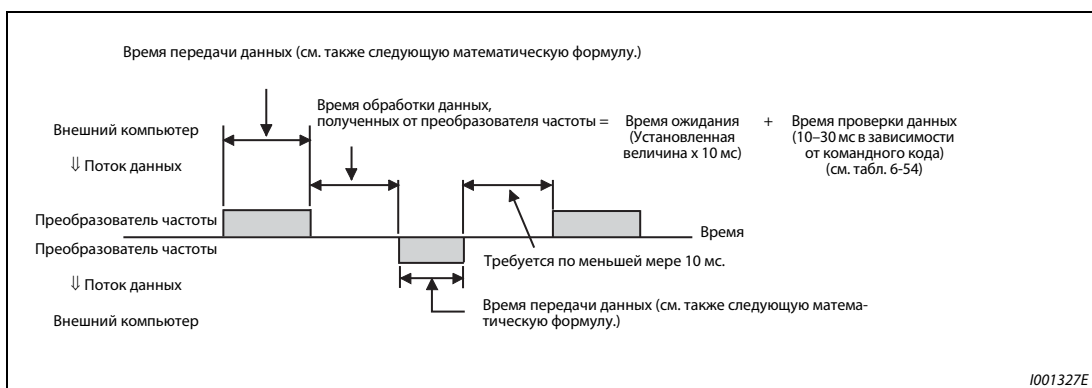
Рис. 6-112: Время передачи данных
