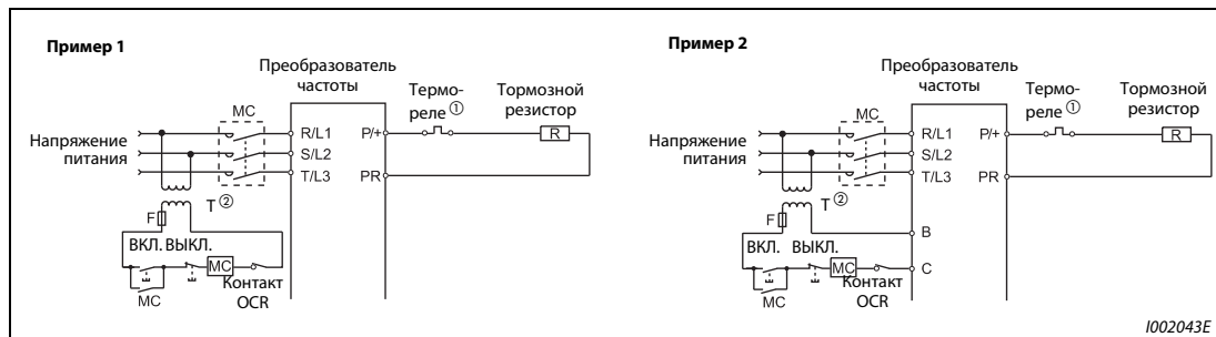
Рис. 3-27: Защитные схемы
