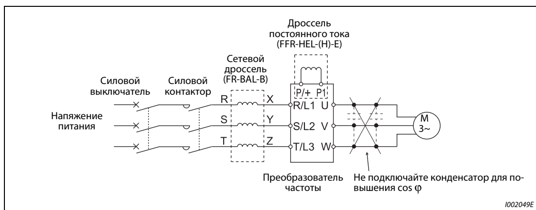
Рис. 3-41: Подавление высокочастотных гармоник в напряжении сети
