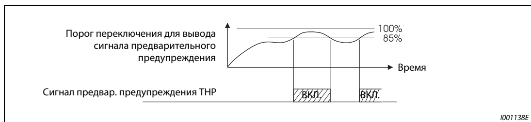
Рис. 6-35: Вывод сигнала предварительного предупреждения
