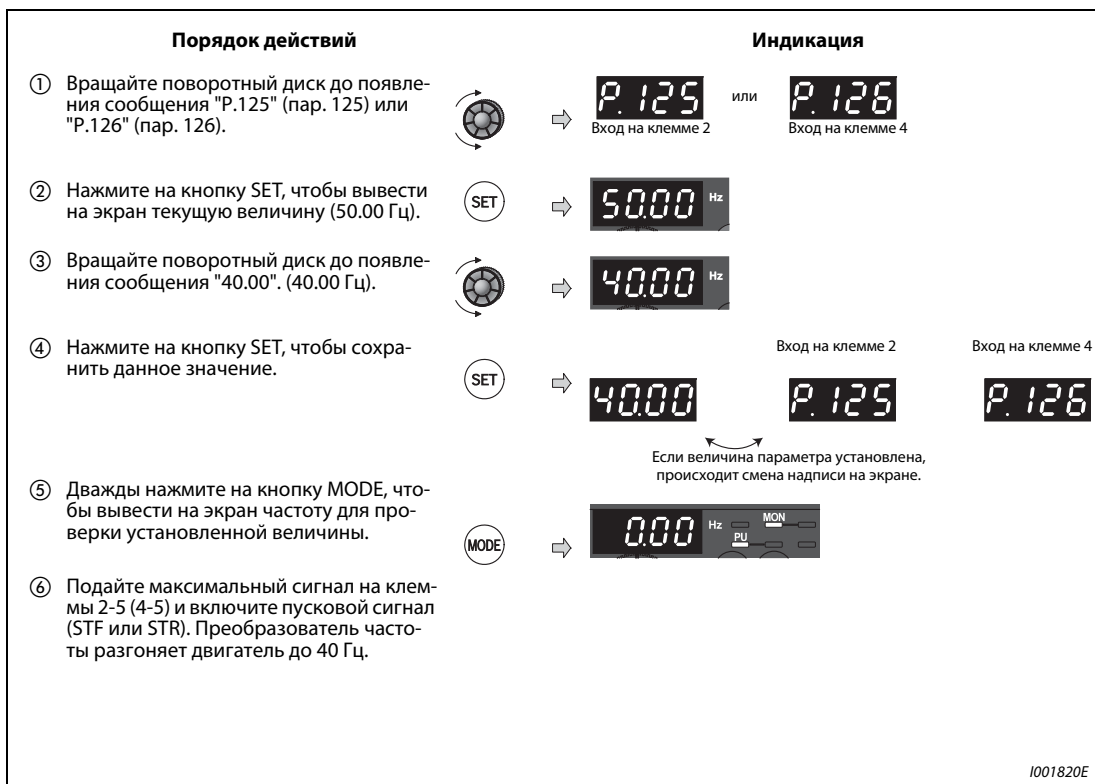
Рис. 6-87: Установка частоты без установки напряжения (тока)
