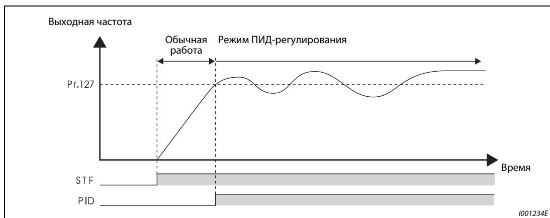
Рис. 6-126: Автоматическое переключение в режим ПИД-регулирования
