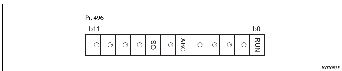
Рис. 6-57: Децентрализованные выходные данные
