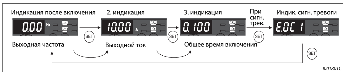
Рис. 6-61: Выбор третьей индикации
