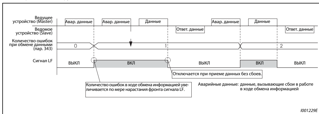
Рис. 6-118: Вывод сигнала LF
