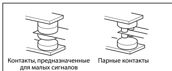
Рис. 3-14: Виды контактов
