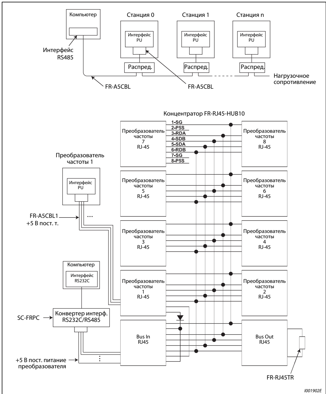
Рис. 6-100: Кабельные соединения с несколькими преобразователями частоты
