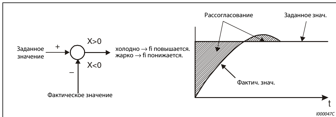
Рис. 6-123: Нагрев
