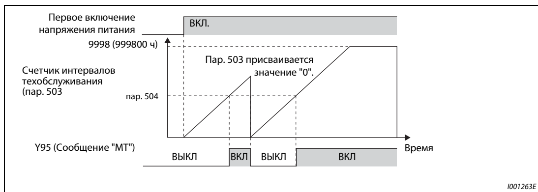
Рис. 6-141: Счетчик интервалов технического обслуживания
