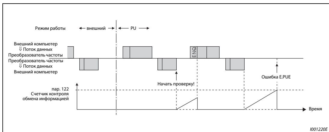
Рис. 6-105: Контроль кабеля на обрыв
