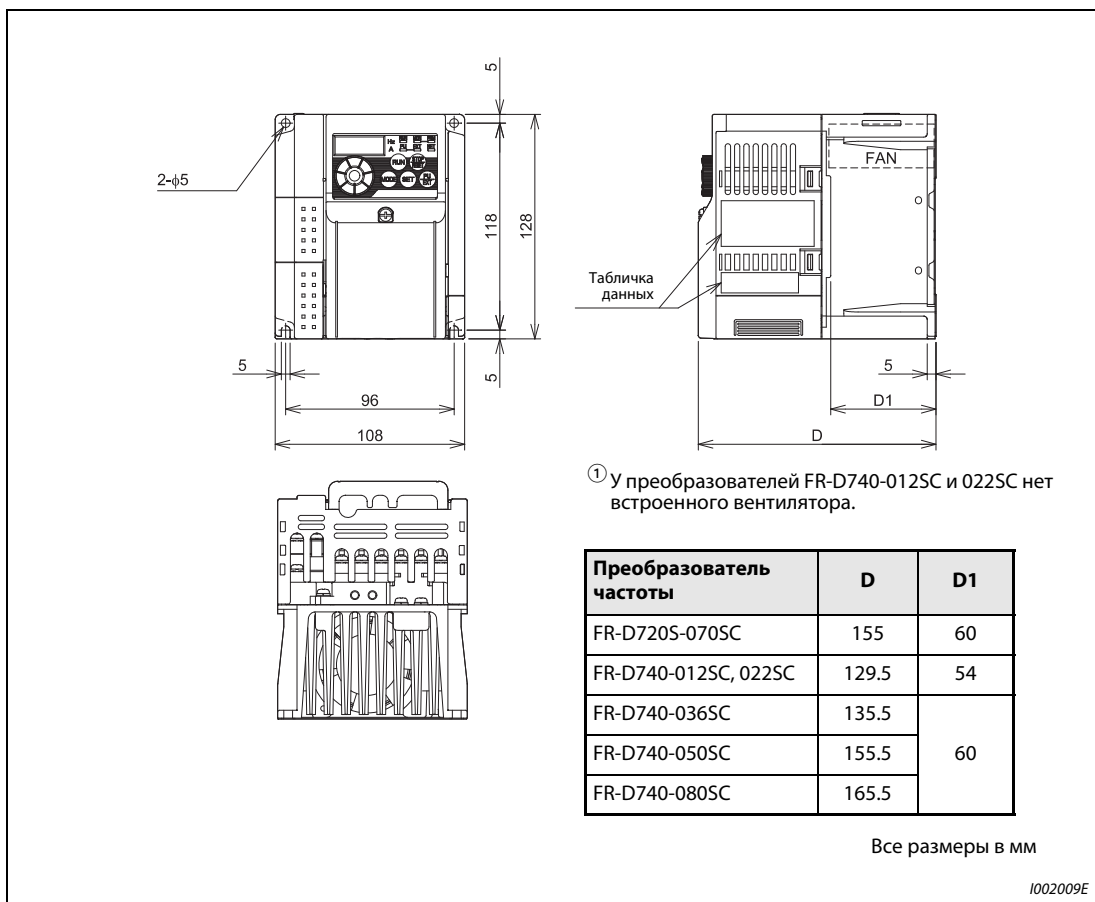
Рис. А-2: Размеры преобразователей частоты FR-D720S-070SC и FR-D740-012SC до 080SC
