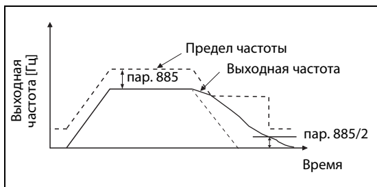
Рис. 6-138: Ограничение выходной частоты
