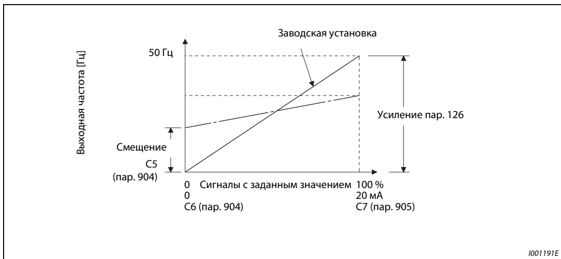
Рис. 6-84: Калибровка сигнала на клемме 4
