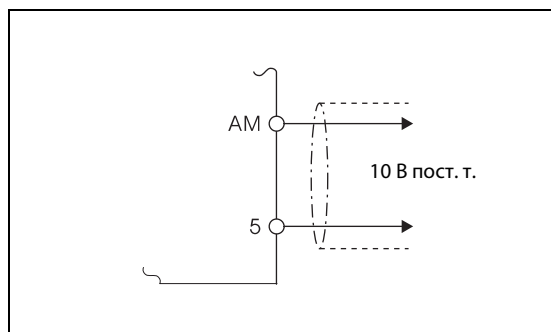
Рис. 6-65: Подключение аналогового индикатора к выходу АМ
