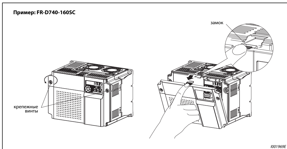
Рис. 2-3: Снятие передней панели
