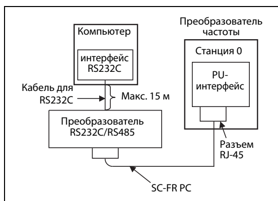
Рис. 6-99: Подключение компьютера с интерфейсом RS232 к интерфейсу PU
