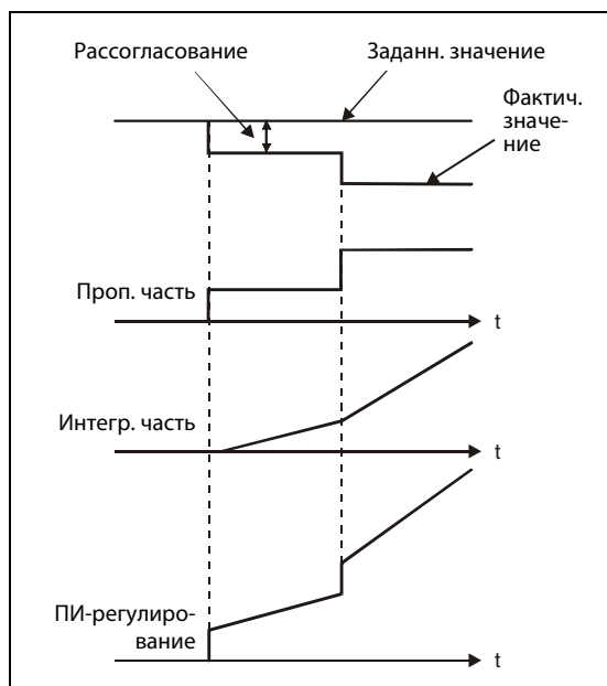
Рис. 6-120: Принцип действия ПИ-регулятора
