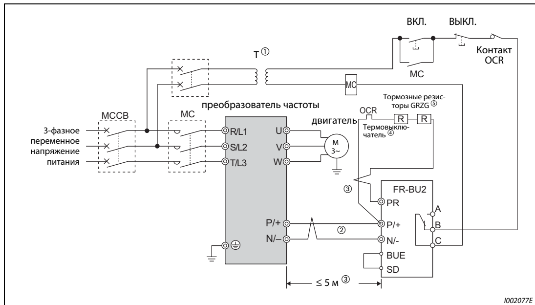
Рис. 3-29: Подключение тормозного устройства типа FR-BU2
