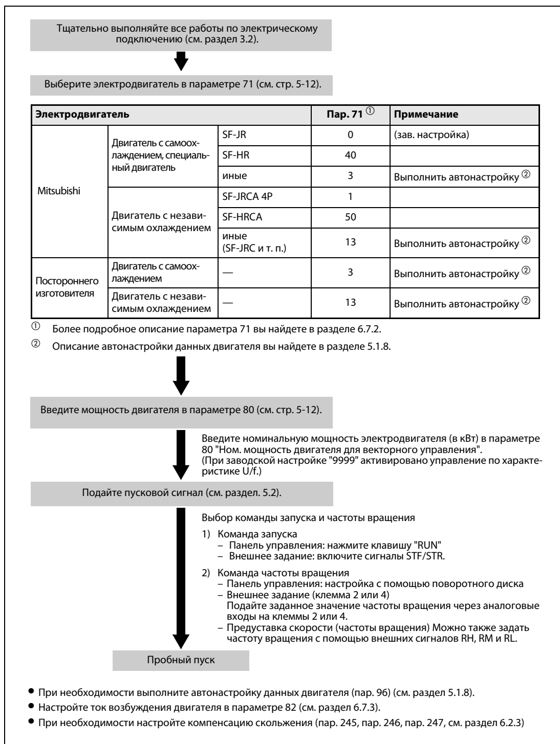
Рис. 6-2: Метод выбора векторного управления
