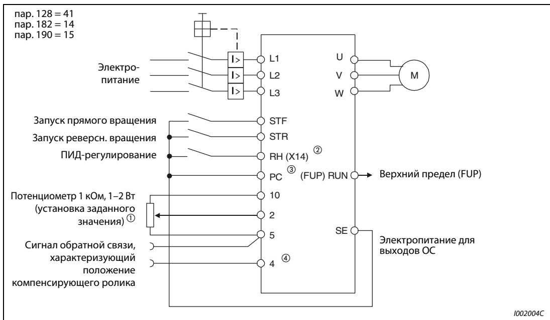
Рис. 6-133: Пример подключения при положительной логике
