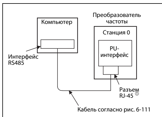
Рис. 6-98: Подключение компьютера с интерфейсом RS485 к интерфейсу PU
