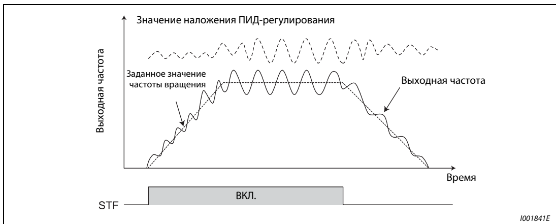
Рис. 6-132: Наложение сигнала при регулировании по положению компенсирующего ролика
