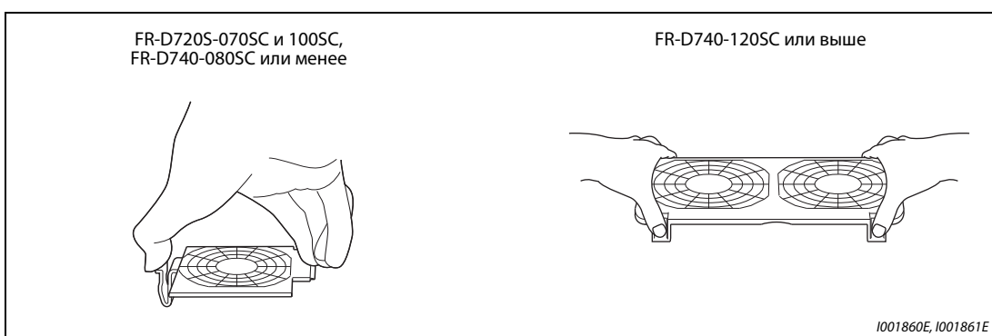
Рис. 8-2: Демонтаж крышки вентилятора
