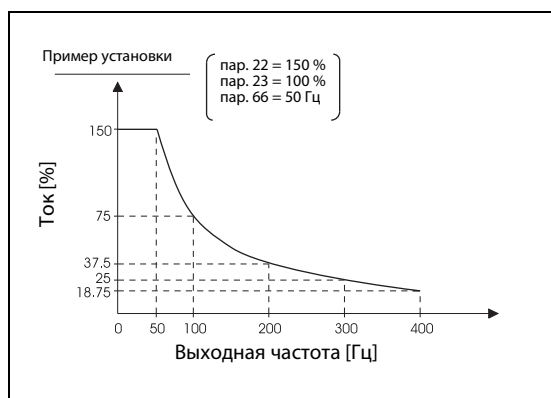
Рис. 6-7: Характеристика предельного тока для пар. 22 = 150 %, пар. 23 = 100 % и пар. 66 = 50 Гц
