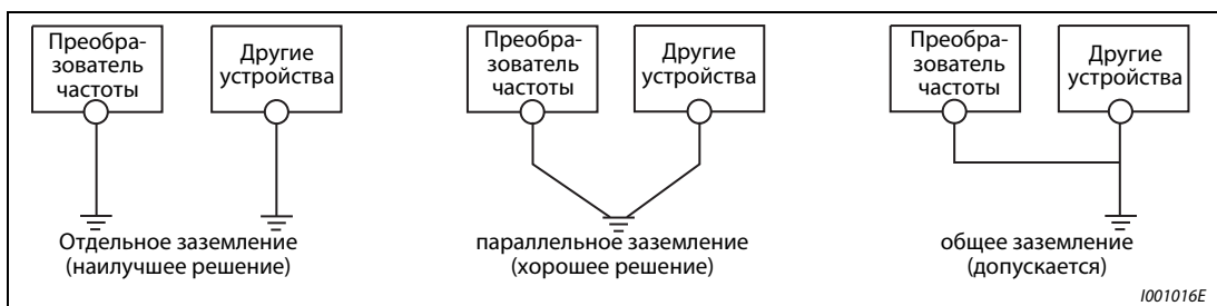
Рис. 3-4: Заземление приводной системы
