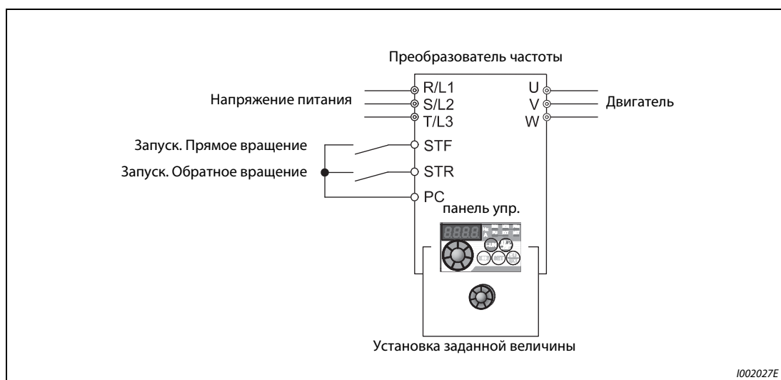
Рис. 5-20: Внешнее управление
