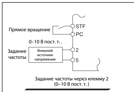
Рис. 6-81: Задание частоты в виде постоянного напряжения 0...10 В
