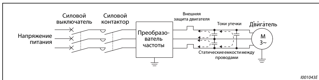
Рис. 3-36: Токи утечки между проводами
