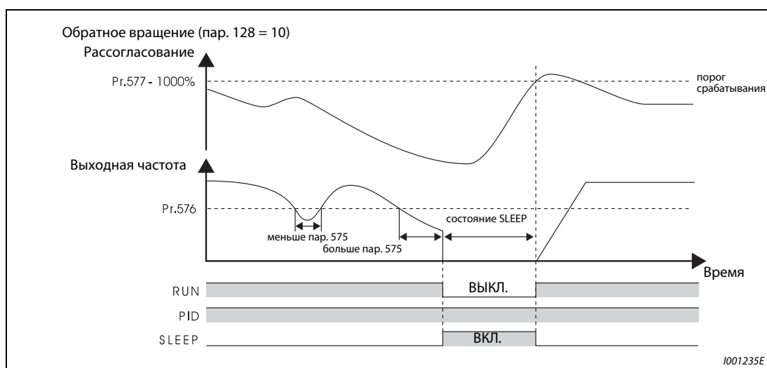
Рис. 6-127: Отключение выхода (функция SLEEP)
