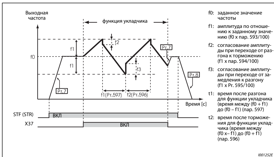
Рис. 6-136: Функция укладчика
