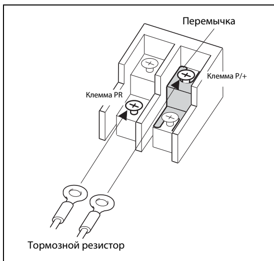
Рис. 3-25: Подключение тормозного резистора к клеммам P/+ и PR преобразователей частоты типов FR-D720S-070SC и 100SC и FR-D740-012SC...080SC
