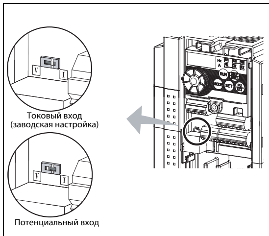
Рис. 6-79: Переключатель "Потенциальный/токовый вход"
