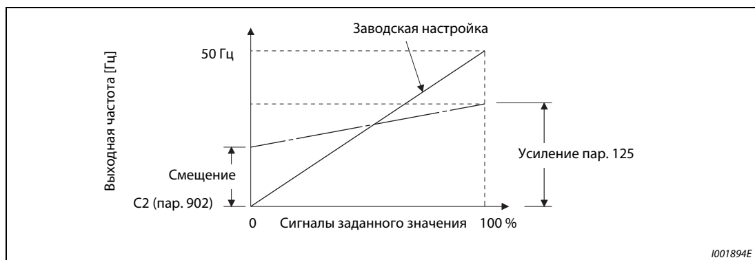
Рис. 6-134: Компенсация сигнала на клемме 2
