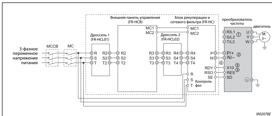
Рис. 3-32: Подключение комбинированного устройства рекуперации энергии/сетевого фильтра FR-HC
