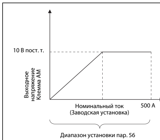
Рис. 6-64: Опорная величина для внешней индикации тока
