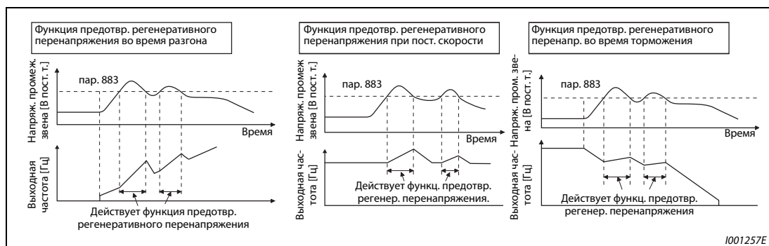
Рис. 6-137: Функция регенеративного перенапряжения.
