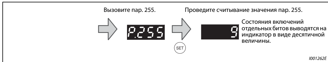
Рис. 6-139: Считывание параметра 255
