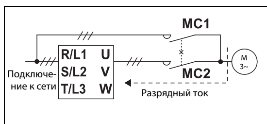
Рис. 4-1: Механическая блокировка силовых контакторов
