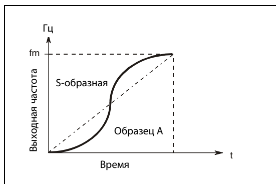
Рис. 6-31: Характеристика при пар. 29 = "1"
