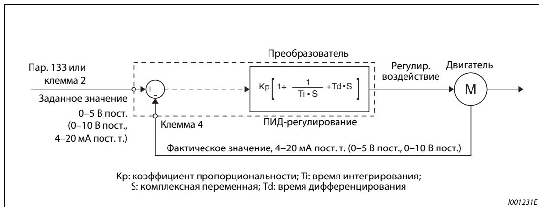
Рис. 6-119: Конфигурация системы для пар. 128 = 20 или 21 подключение задания/сигнала обратной связи к преобразователю)
