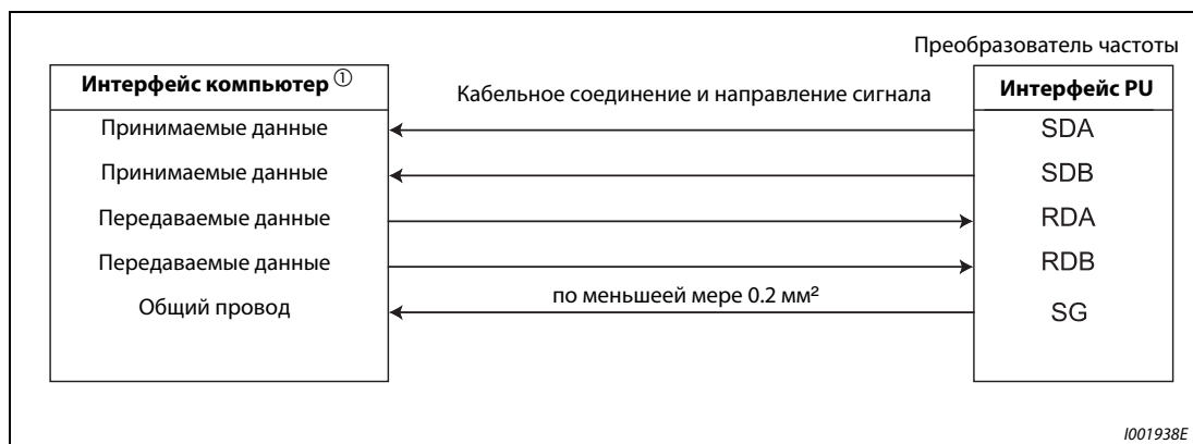
Рис. 6-101: Кабельное соединение с преобразователем частоты
