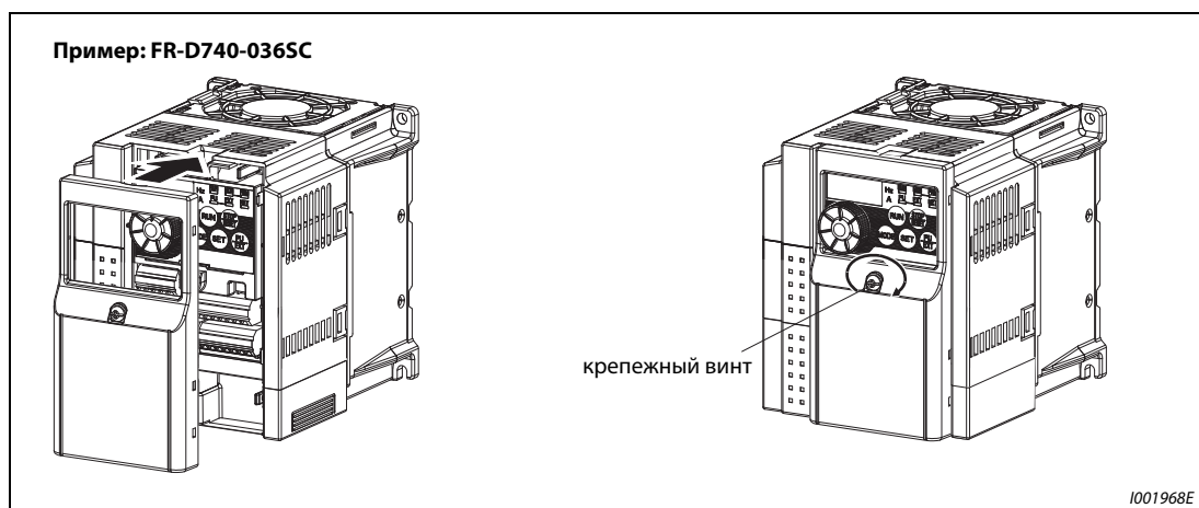
Рис. 2-2: Установка передней панели
