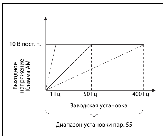
Рис. 6-63: Опорная величина для внешней индикации частоты
