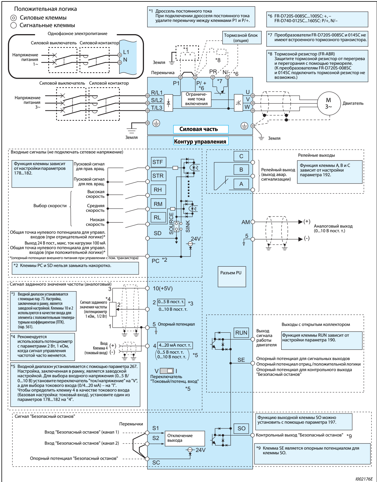
Рис. 3-3: Схема подключения преобразователя частоты
