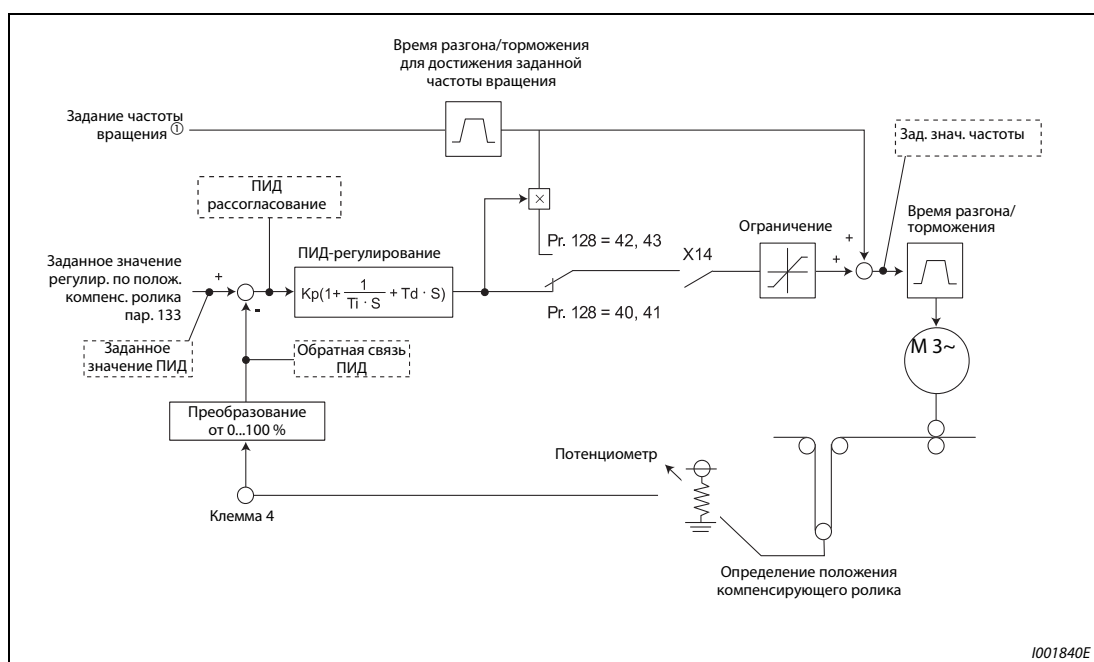
Рис. 6-131: Блок-схема регулирования по положению компенсирующего ролика (танцующего потенциометра)
