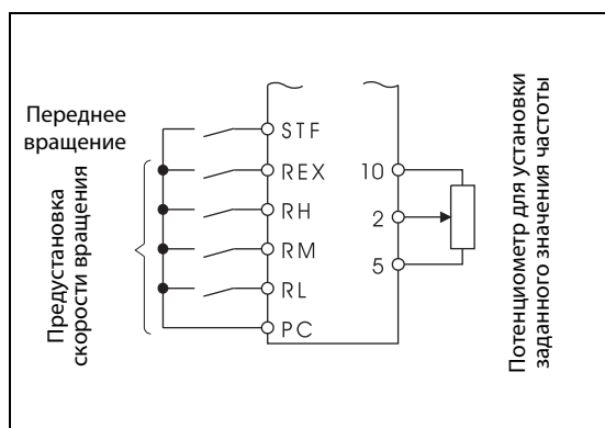
Рис. 6-17: Пример подключения
