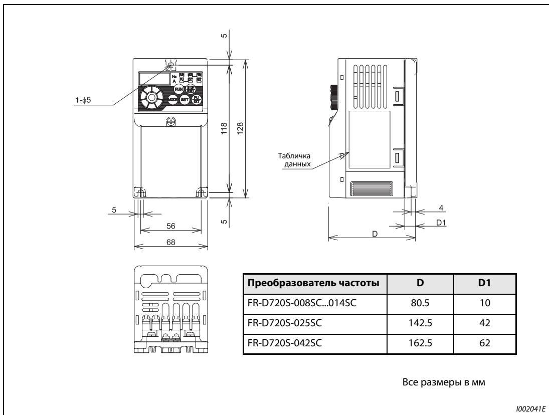
Рис. А-1: Размеры преобразователей частоты FR-D720-008SC...042SC
