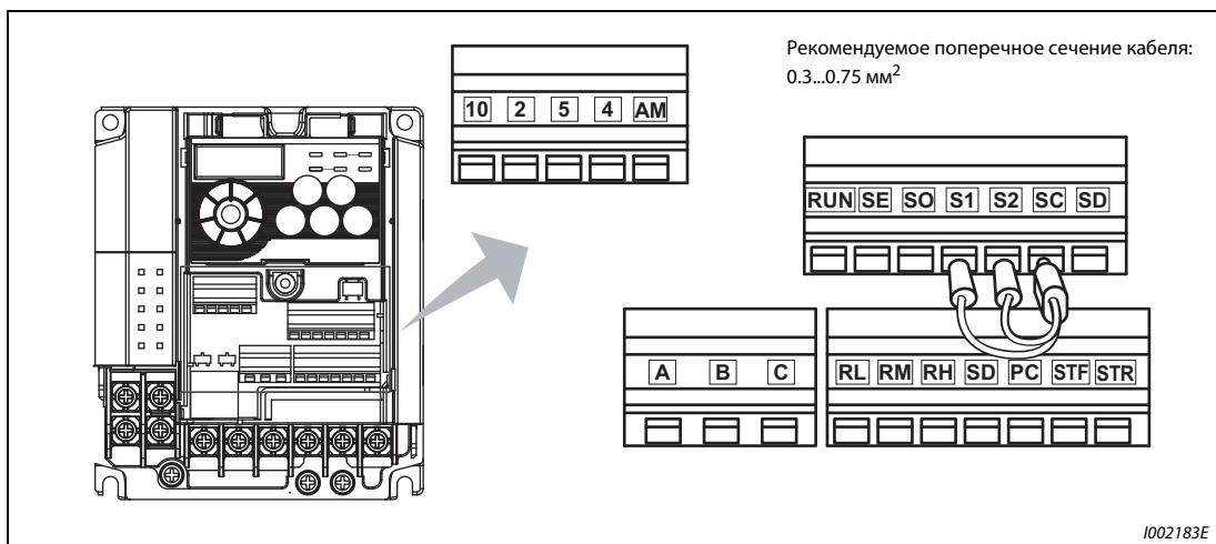
Рис. 3-6: Расположение клемм
