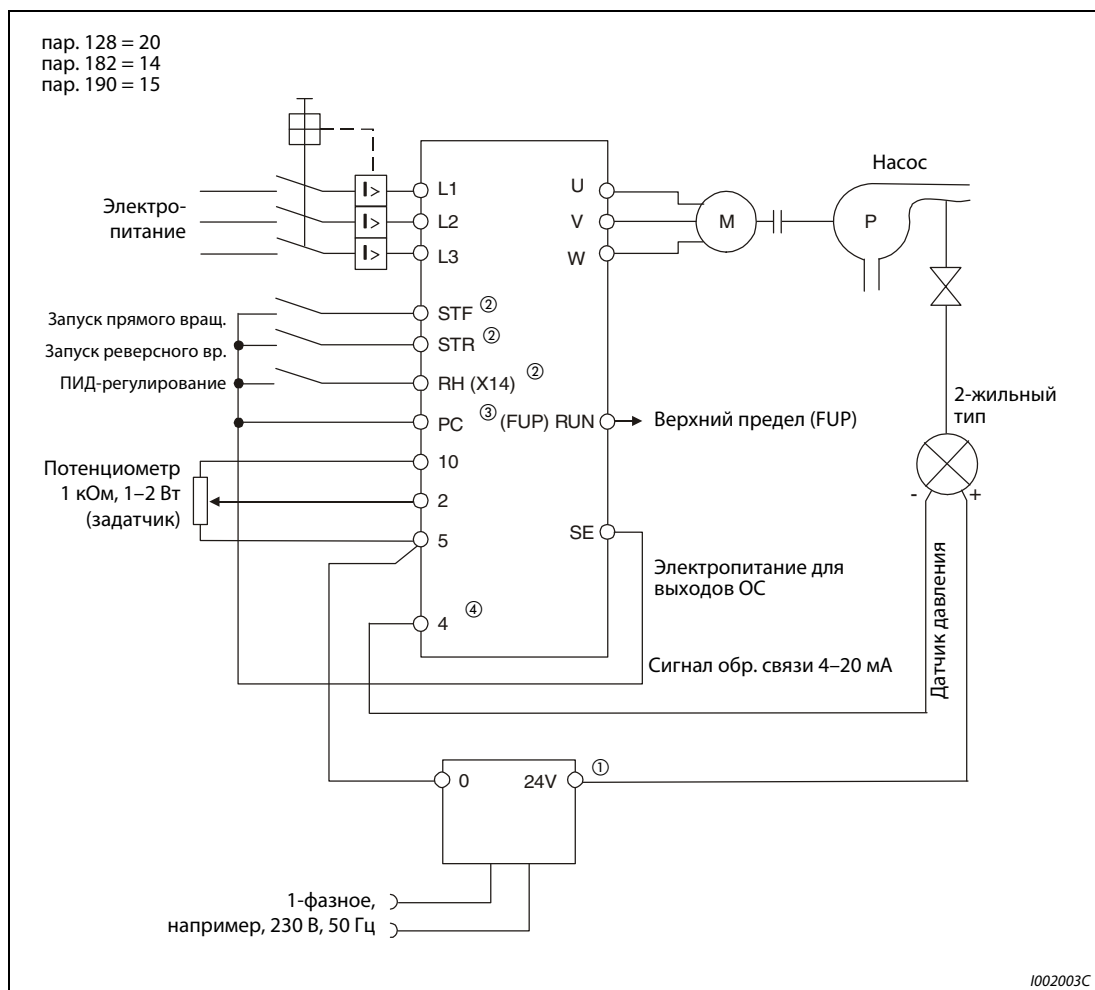
Рис. 6-125: Пример подключения при положительной логике
