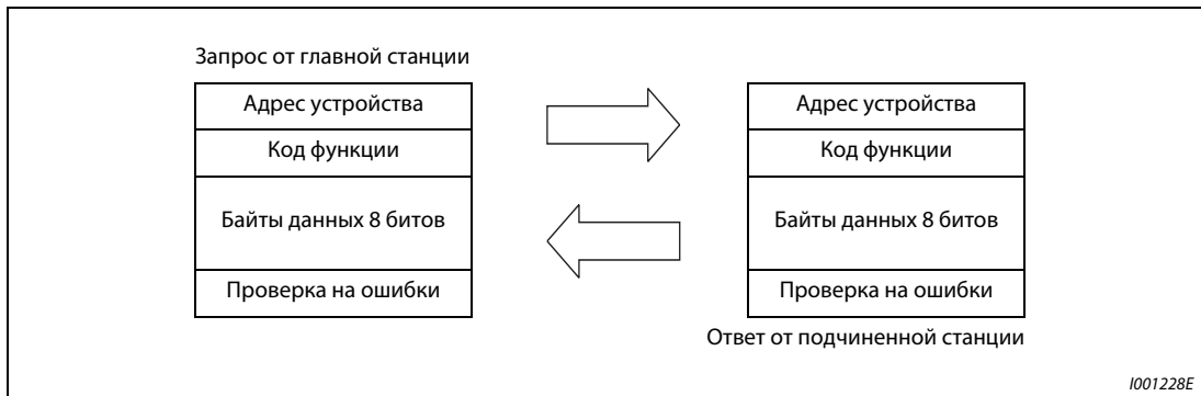
Рис. 6-117: Обмен данными
