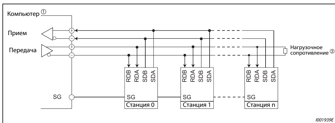
Рис. 6-102: Соединение с несколькими преобразователями частоты
