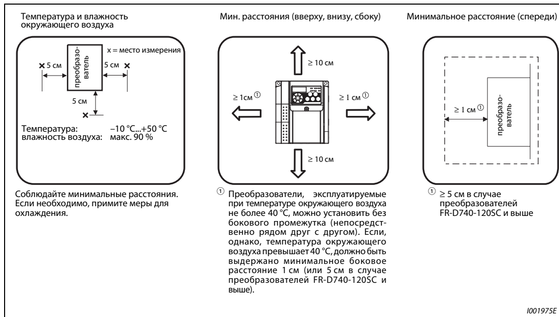
Рис. 2-9: Минимальные зазоры
