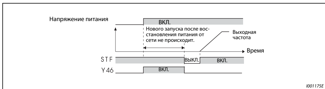
Рис. 6-73: Новый запуск при восстановлении питания
