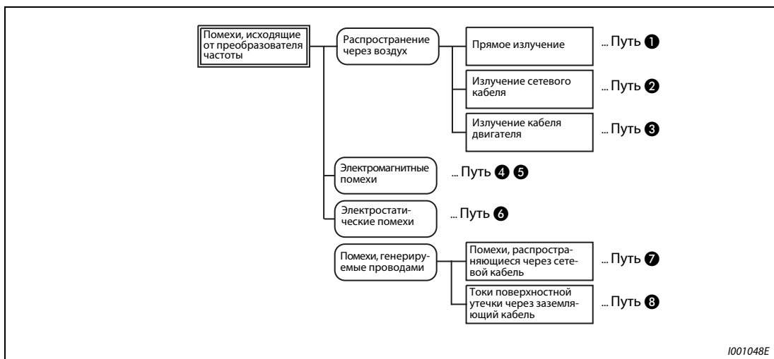
Рис. 3-38: Распространение помех
