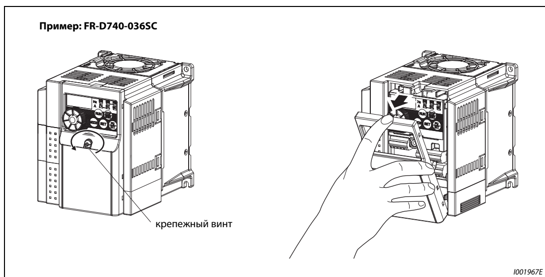
Рис. 2-1: Снятие передней панели
