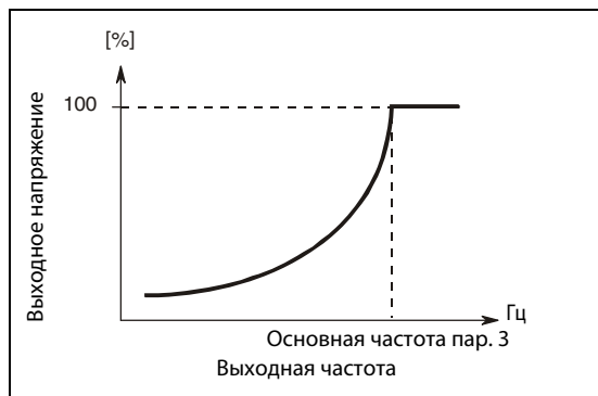
Рис. 6-13: Квадратичная характеристика
