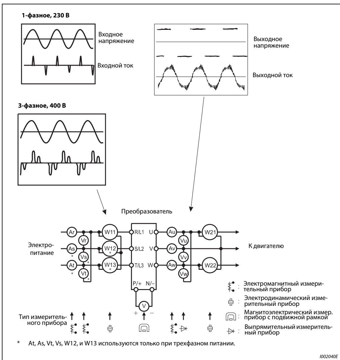
Рис. 7-7: Измерения на силовой части
