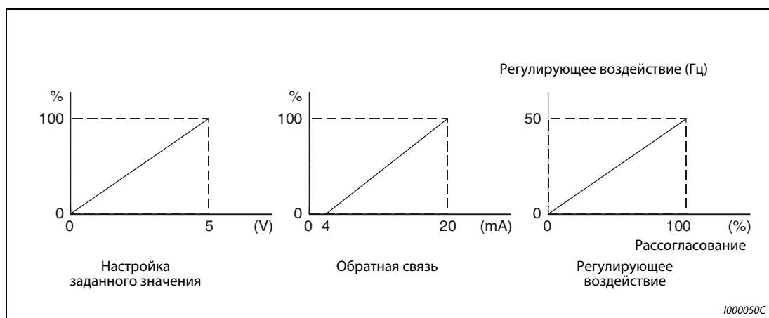
Рис. 6-130: Калибровка входов
