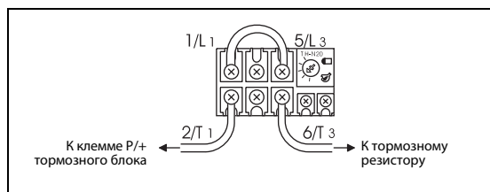
Таб. 3-20: Комбинация тормозного резистора GRZG и термореле
