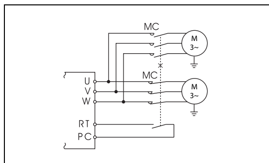
Рис. 6-34: Питание двух двигателей от одного преобразователя частоты
