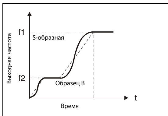
Рис. 6-32: Характеристика при пар. 29 = "2"
