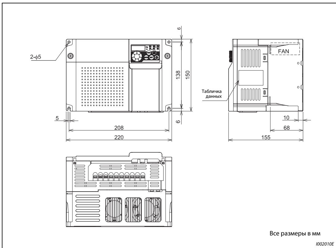
Рис. А-4: Размеры преобразователя частоты FR-D740-120SC и 160SC
