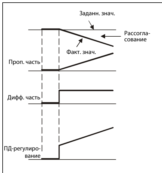
Рис. 6-121: Принцип действия ПД-регулятора
