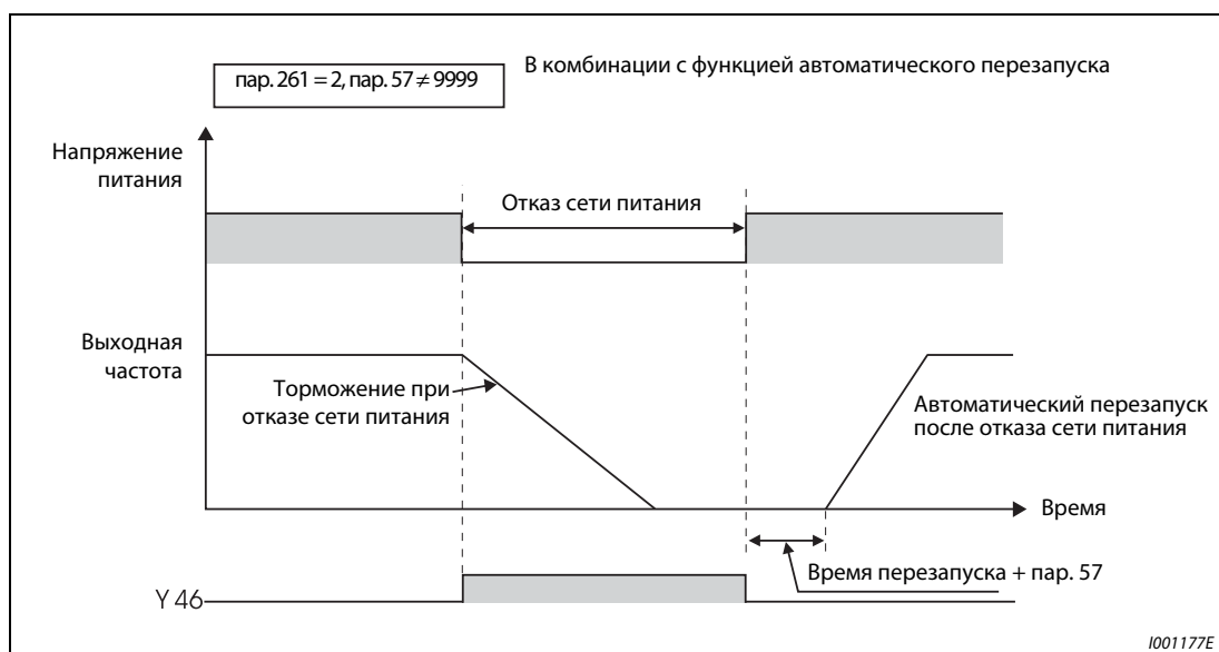
Рис. 6-75: Продолжение работы после отказа сети
