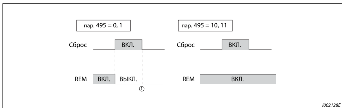
Рис. 6-59: Данные децентрализованного вывода при сбросе преобразователя частоты
