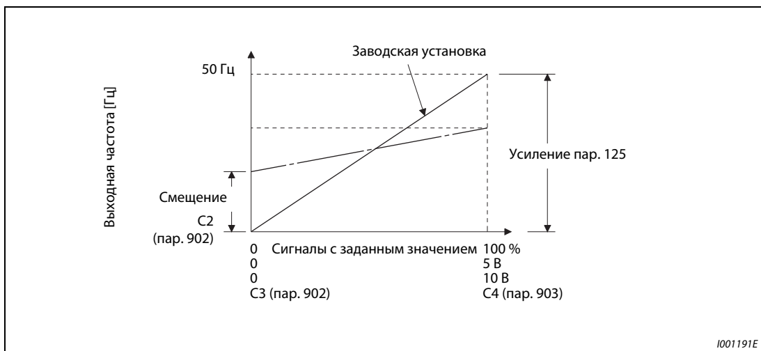
Рис. 6-83: Калибровка сигнала на клемме 2
