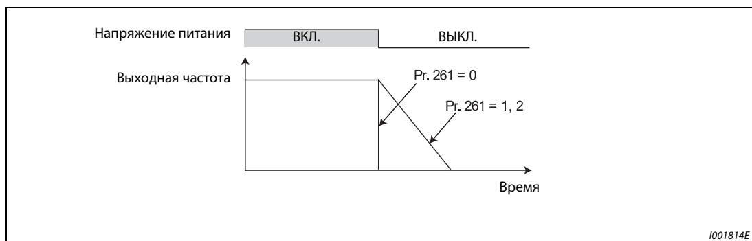
Рис. 6-71: Параметры для выбора способа останова при отказе сети питания
