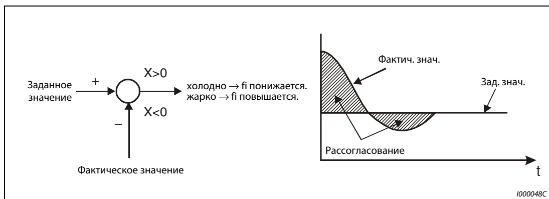
Рис. 6-124: Охлаждение
