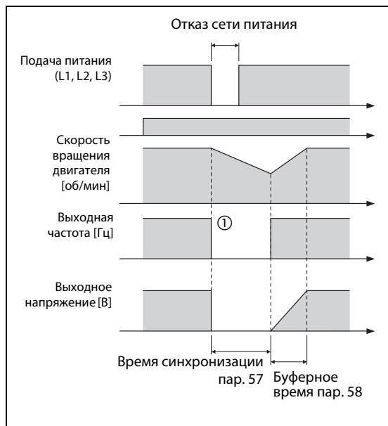
Рис. 6-68: Автоматический перезапуск без определения выходной частоты (пар. 162 = 1/11)
