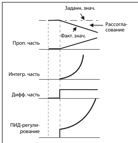
Рис. 6-122: Принцип действия ПИД-регулятора
