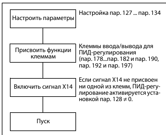
Рис. 6-128: Метод настройки
