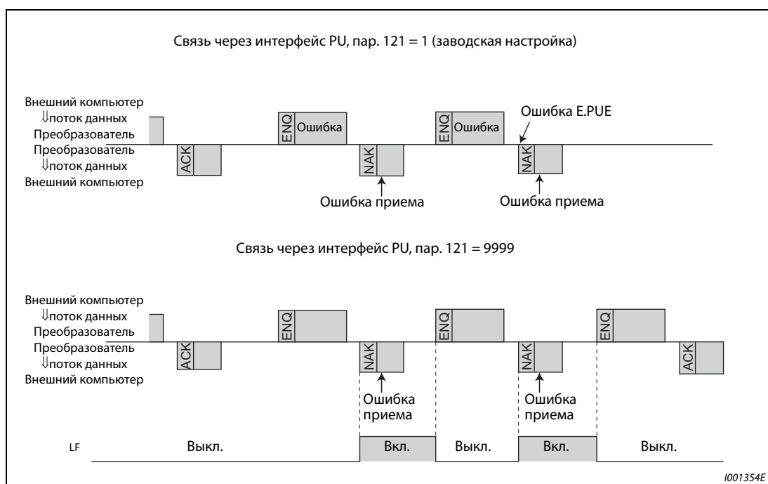
Рис. 6-104: Ошибки передачи данных
